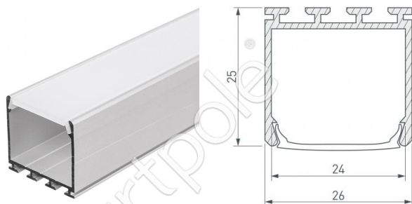
1 Световой профиль Артикул: 006123 Размер: 2000x26x25 мм
